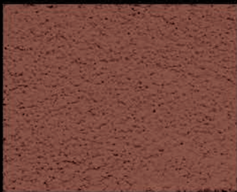
TANZANITE
