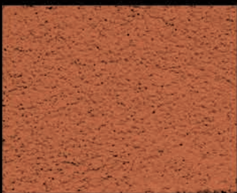
CURITE
